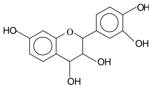
FLAVAN-3,4-DIOL
